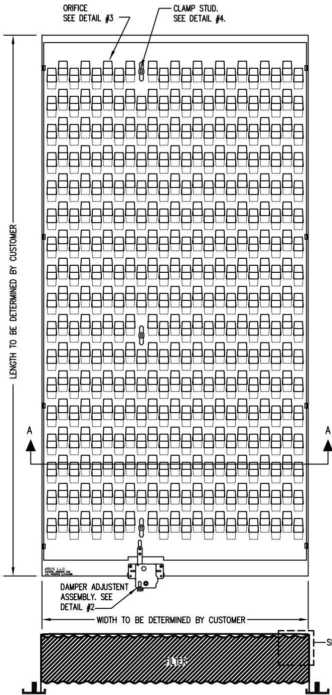
SECTION A-A
