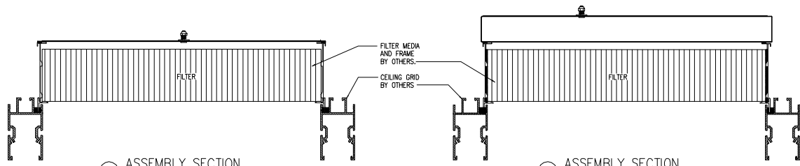
② B ASSEMBLY SECTION SCALE: 1:3
