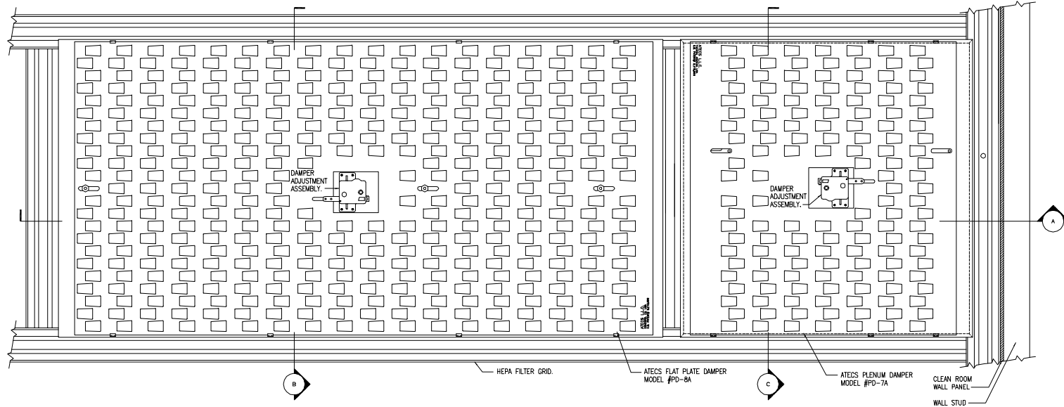
① PLENUM ASSEMBLY - TOP VIEW SCALE: 1:3
