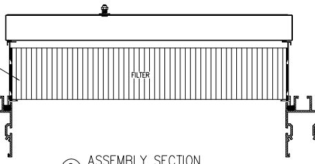
C ASSEMBLY SECTION SCALE: 1:3
