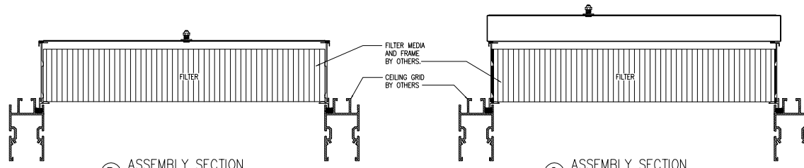
B ASSEMBLY SECTION SCALE: 1:3
